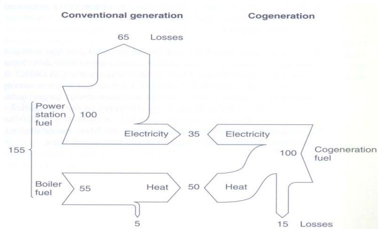
شکل ۴-۷- مقایسه یک واحد CHP با نوع متداول
