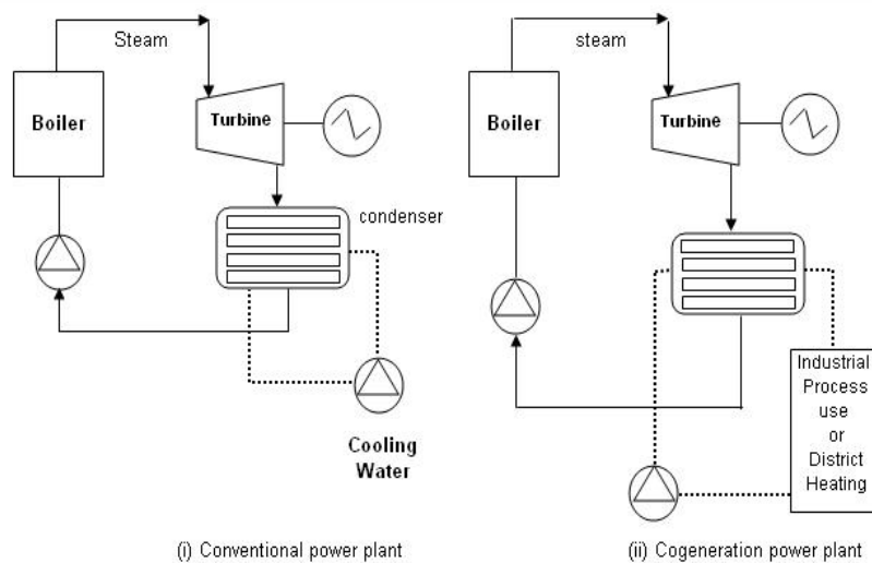
شکل ۴-۱۰- نمودار شماتیک نیروگاه تولید مشترک و متداول
