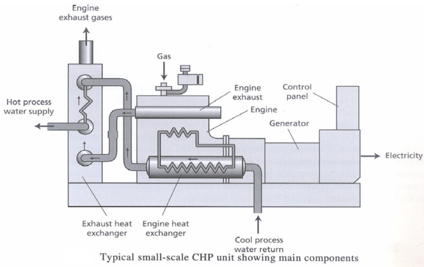
شکل ۴-۶- نوعی سیستم تولید مشترک برق و حرارت که مؤلفه‌های اصلی را نشان
